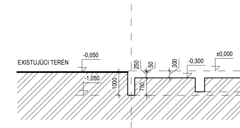
REZ A-A
